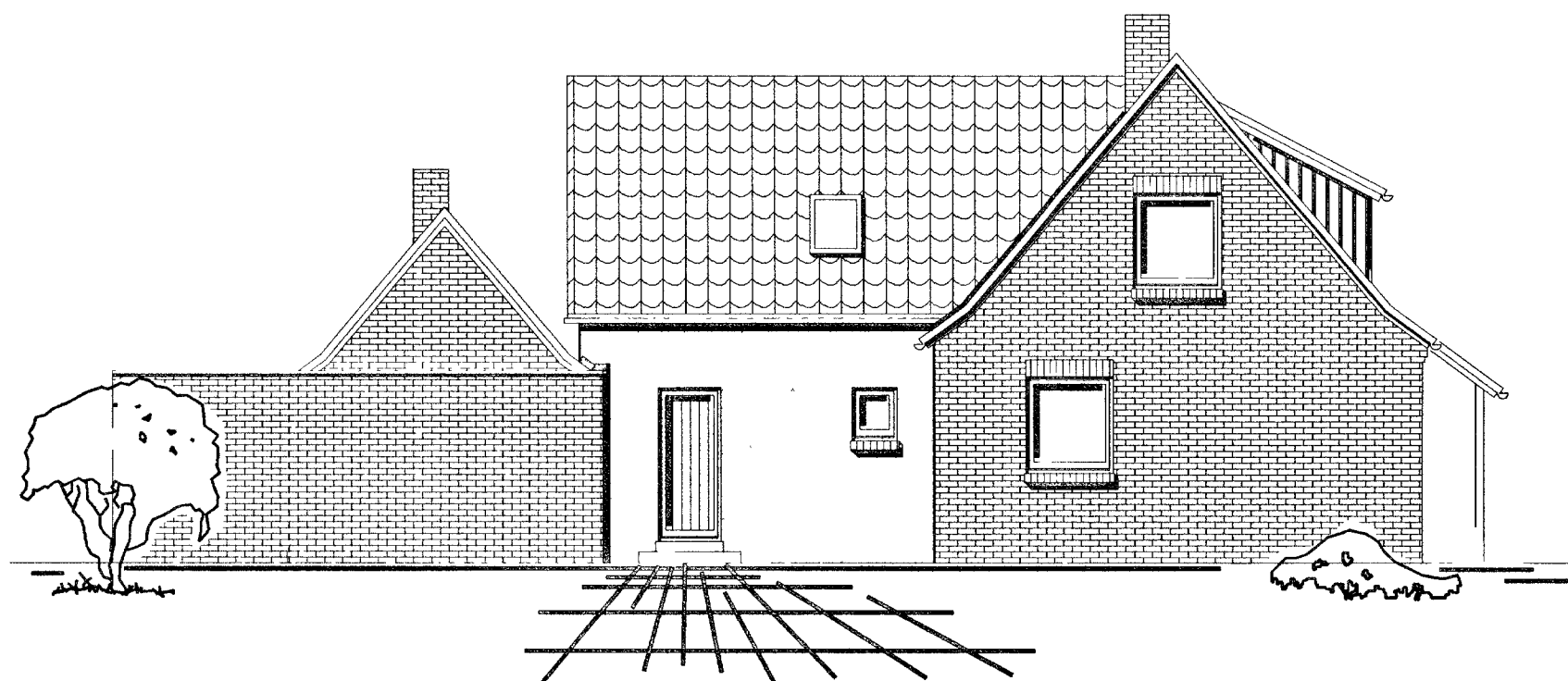
Nord - Ansicht
